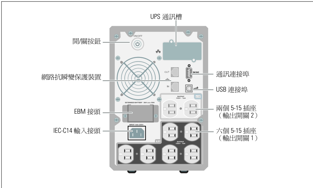
圖 5. 1000W，120V 後面板
