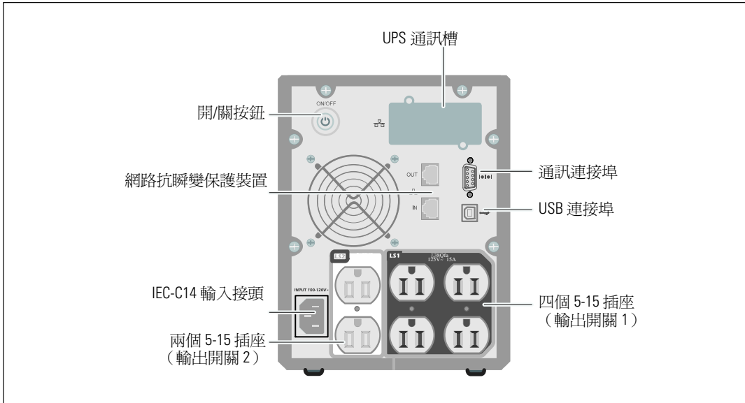
圖 3. 500W，100/120V 後面板
