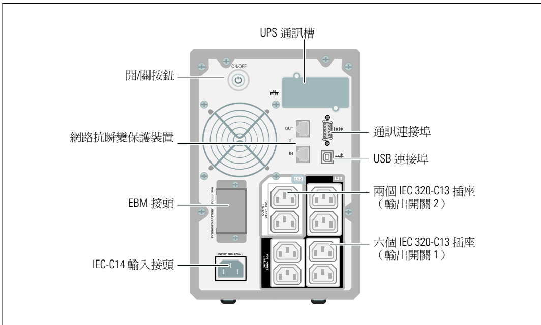
圖 6. 1000W，230V 後面板
