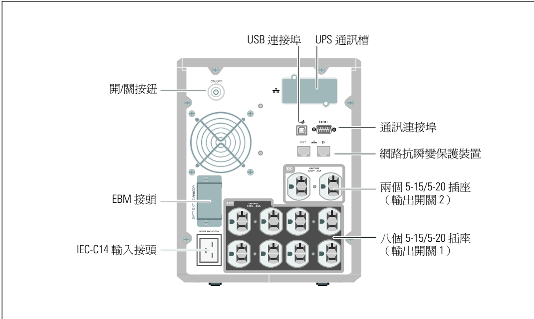
圖 7. 1920W/120V, 1500W/100V 後面板
