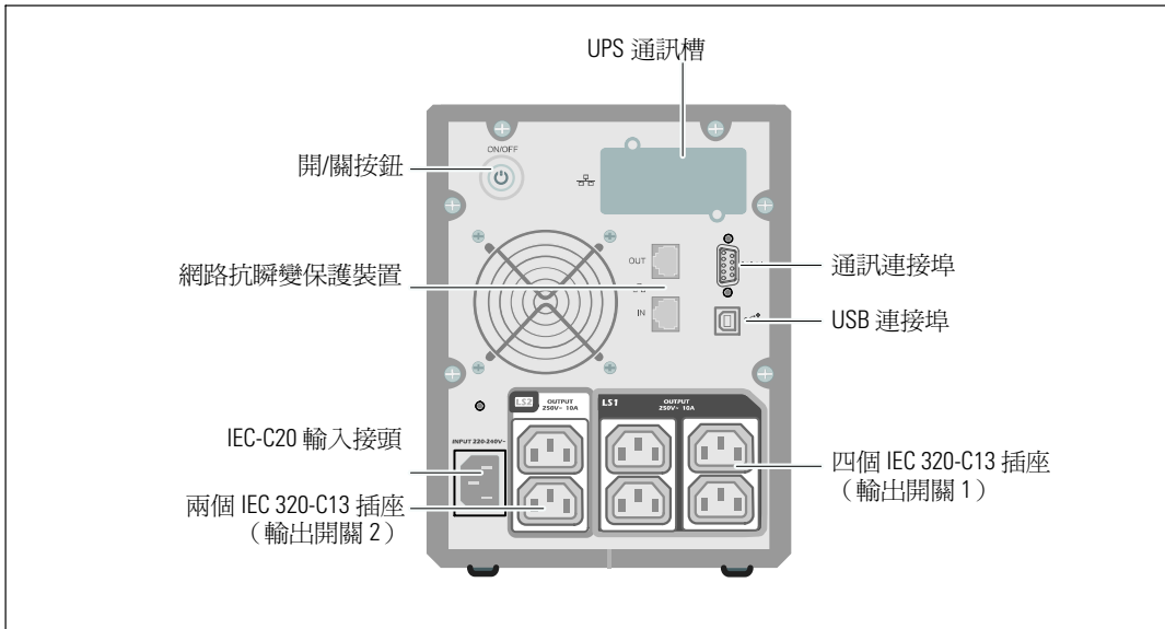
圖 4. 500W，230V 後面板
