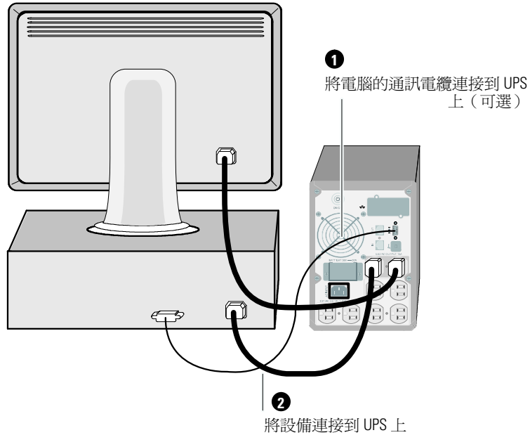
圖 16. 典型的 UPS 安裝（示出的為 120V 型號）
