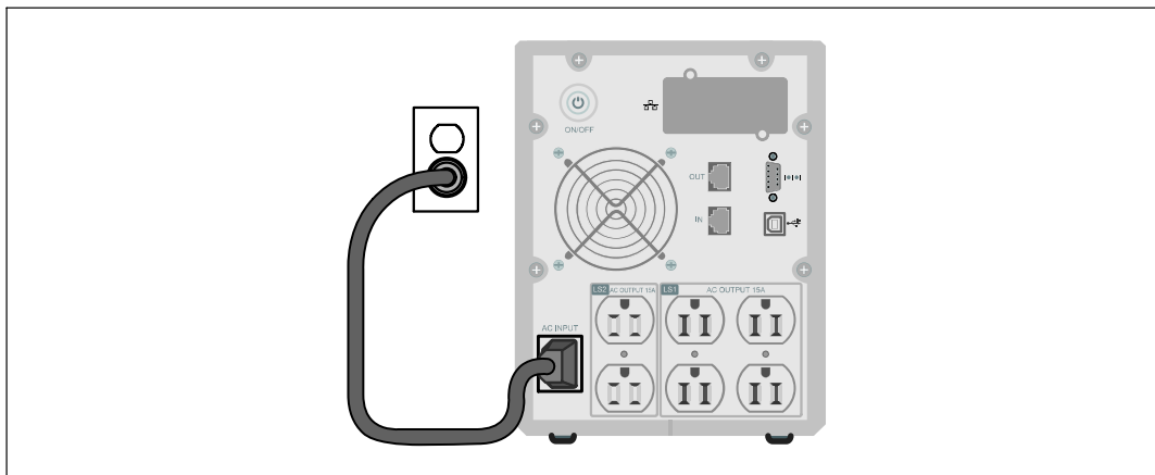
圖 17. 連接電源線
