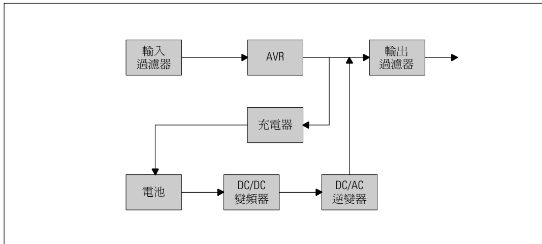
圖 27. 在線互動式 UPS 區塊圖
