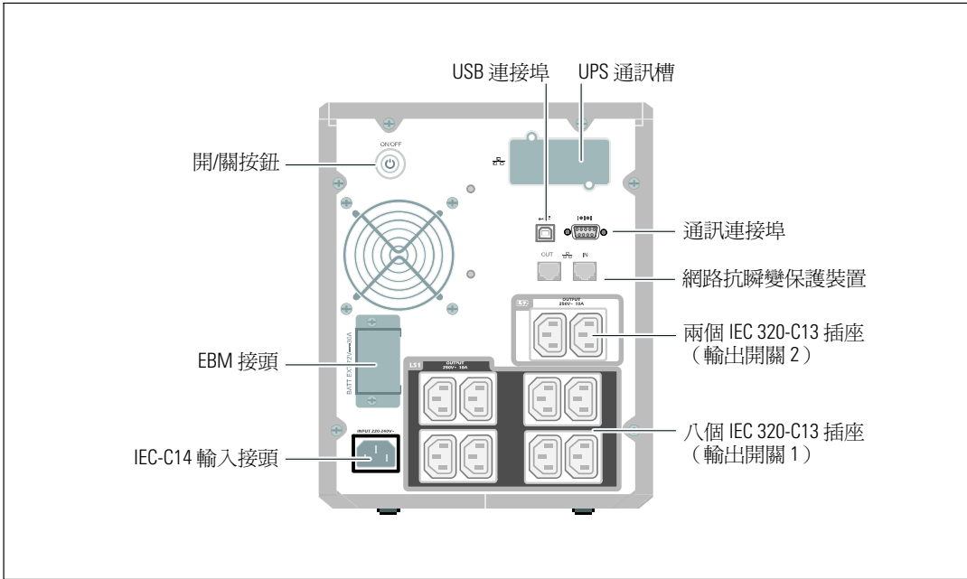
圖 8. 1920W, 230V 後面板
