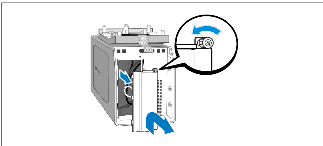
圖 11. 取下電池蓋
