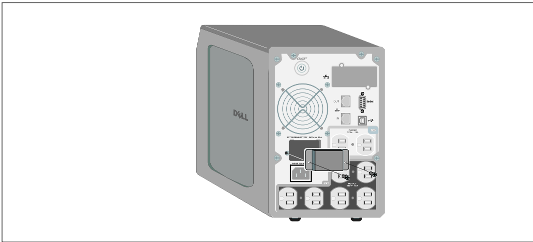
圖 13. 取下電池接頭蓋
