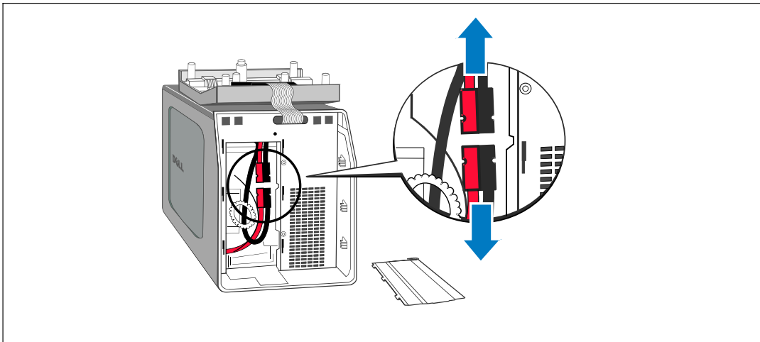
圖 26. 斷開 UPS 內置電池連接器
