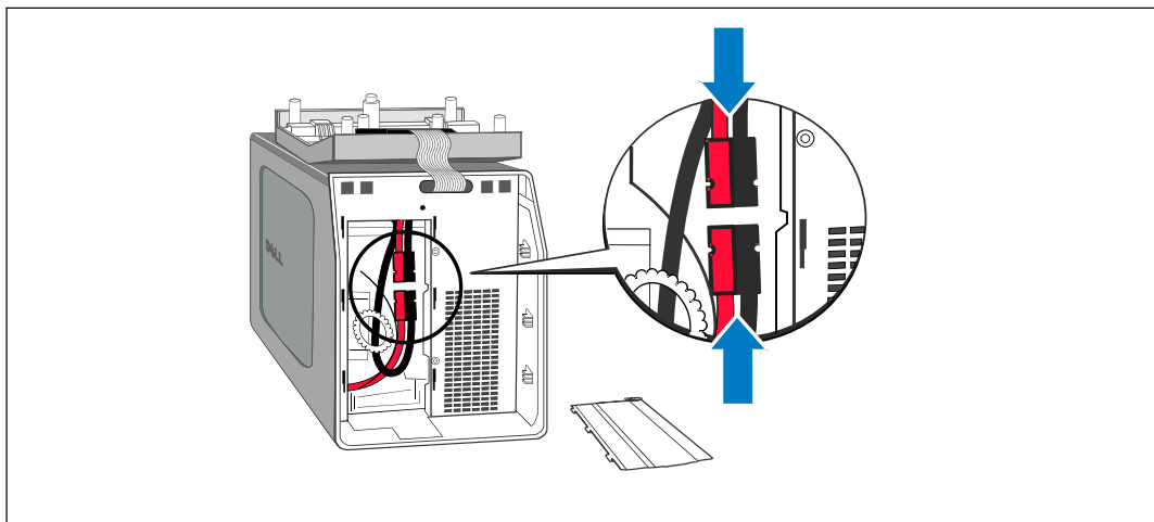
圖 12. 連接內置電池接頭
